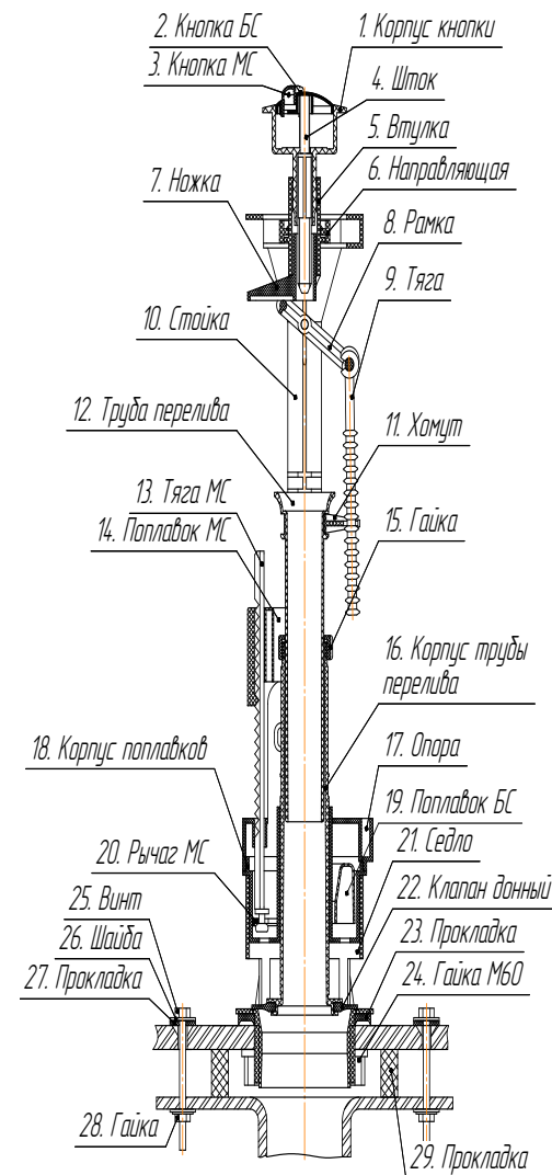
Рис.2 Клапан выпуска.
