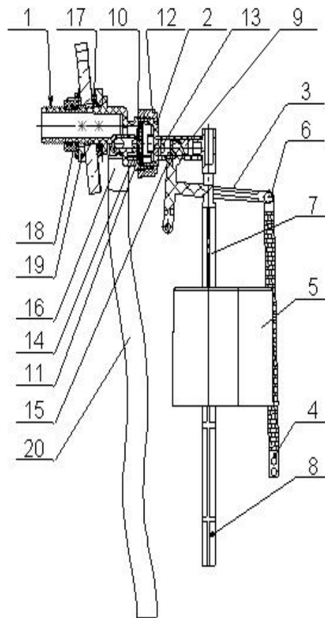
Рис.1 Клапан наполнительный.
